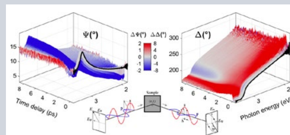
Obr. 159 Časová evoluce eliptometrických úhlů \Psi (amplitudový poměr) a \Delta (fázový rozdíl) tenkého filmu ZnO po nerezonantním UV vybuzení měřeném při 60^\circ úhlu dopadu. Přírůstky vzhledem k počátečnímu spektru před excitací (černá) jsou zobrazeny modře, poklesy červeně. Schéma v dolní části ilustruje význam eliptometrických parametrů.
