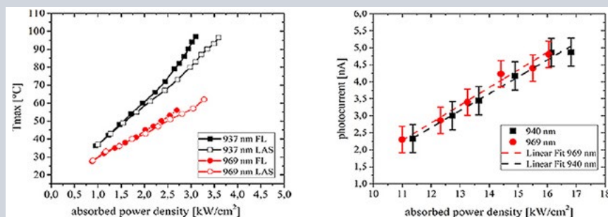
Obr. 121 (a) Teplota povrchu Yb:YAG krystalu měřená termokamerou pro buzení na vlnových délkách 940 a 969 nm; (b) indukovaný fotoproud měřený pikoampérmetrem pro obě budící vlnové délky.
