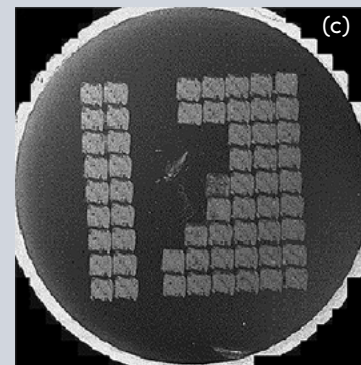
Obr. 128 (a) Čočka teleskopu poškozená zmenšeným top-hat svazkem; (b) Prostorový profil svazku systému Bivoj po zmenšení na 3 \times 3 \text{ mm}^2 ; (c) Vzorek skla s AR nanostrukturou po testu na práh poškození top-hat svazkem.
