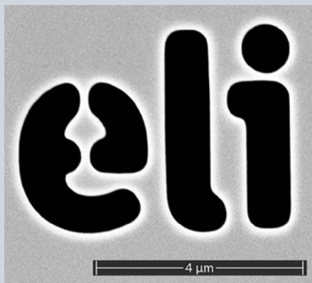
Obr. 154 Obrázek objektu v rastrovacím elektronovém mikroskopu (vlevo). Rekonstrukce obrazu tohoto objektu osvětleného 21. harmonickou frekvencí Ti:S laseru s vlnovou délkou 38 nm (vpravo).
