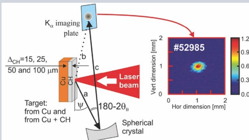
Obr. 145 Schéma diagnostiky horkých elektronů založené na principu dvoudimenzionálního zobrazování rentgenové emise z terčů obsahujících Cu. Typická experimentální data demonstrují distribuci horkých elektronů na povrchu laserem ozářeného vrstevnatého terče.
