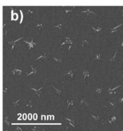
Obr. 50: Schéma heterogenní katalýzy křemíkových nanodrátů v silanovém plazmatu (vlevo) a závislost pravděpodobnosti nukleace (a) ilustrovaná snímky z elektronového mikroskopu (b) a (c) pro různou hustotu kovových zárodků.
