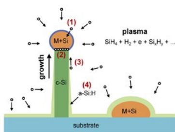
Obr. 50: Schéma heterogenní katalýzy křemíkových nanodrátů v silanovém plazmatu (vlevo) a závislost pravděpodobnosti nukleace (a) ilustrovaná snímky z elektronového mikroskopu (b) a (c) pro různou hustotu kovových zárodků.
