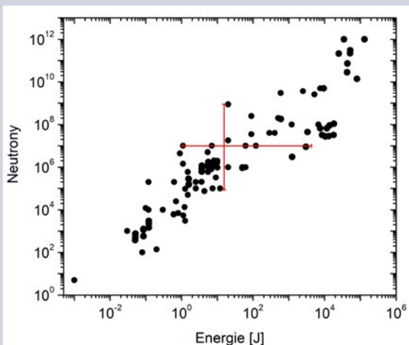
Obr. 143 Zisk fúzních neutronů z deuterovaných terčů ozářených různými laserovými systémy v závislosti na deponované laserové energii.
