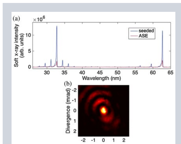
Obr. 155 Spektrum dvoubarevného Kr rentgenového laseru fungujícího na principu ASE a spektrum zesílených harmonických injektovaných do tohoto plazmatu (a) a intenzitní profil takto generovaného XUV svazku (b).
