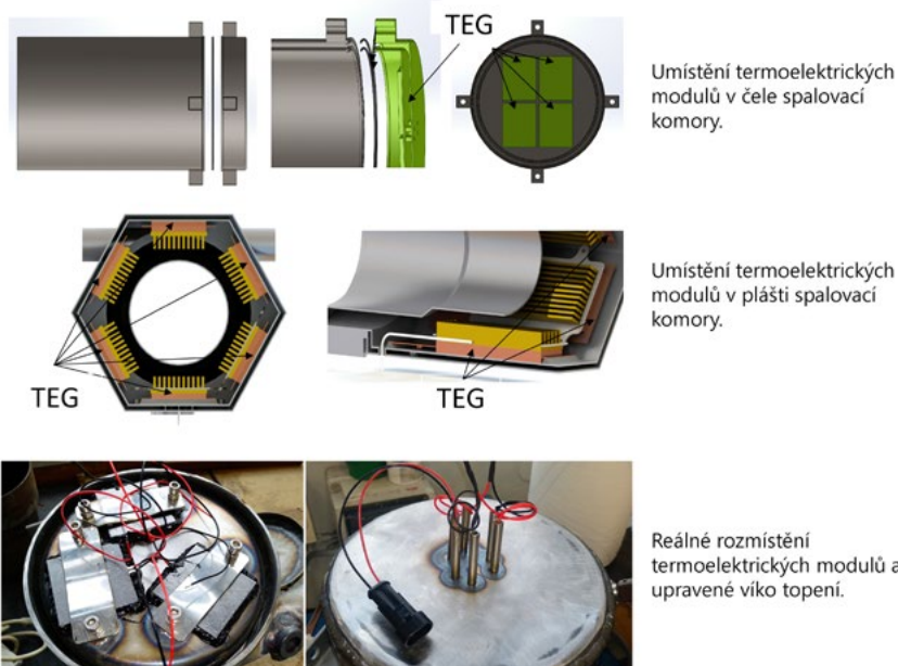
Obr. 48: Nákrasy dvou navržených možností a reálné umístění termoelektrických modulů v nezávislém topení.
