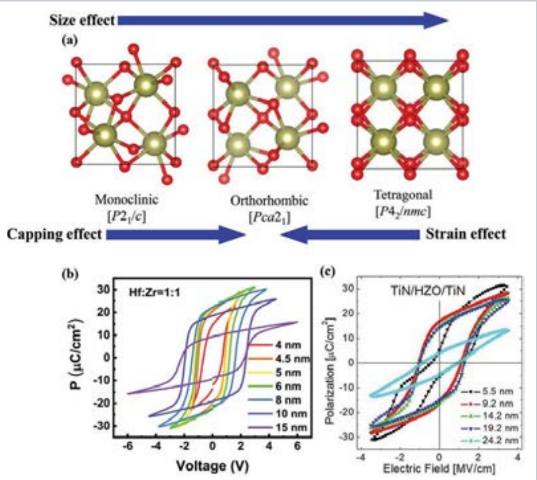
Obr. 2.2.2 Závislost krystalové struktury HfO 2 na tloušťce tenké vrstvy, mechanickém napětí a elektrodách. (a) (100) projekce HfO 2 struktury v monoklinické, ortorombické a tetragonální fázi. Vývoj objemově stabilní monoklinické do výše symetrické tetragonální a feroelektrické ortorombické fáze ilustruje vliv objemového a povrchového efektu, který preferuje vyšší symetrii. Jak povrchová energie, tak i deformace pnutím stabilizuje narušení centra symetrie ve feroelektrické fázi. (b) Polarizační hysterezní smyčky Hf 1-x Zr x O 2 s poměrem Hf:Zr = 1:1 při různých tloušťkách vrstev a s různými elektrodami.
