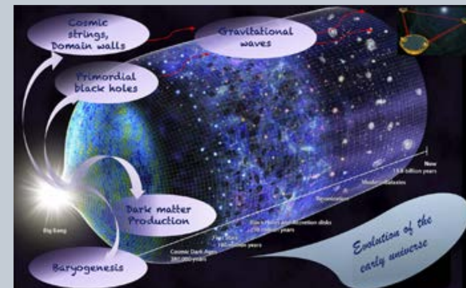
Obr. 2.1.4 Vývoj vesmíru a propagace gravitačních vln z událostí v ranných fázích vývoje vesmíru.
