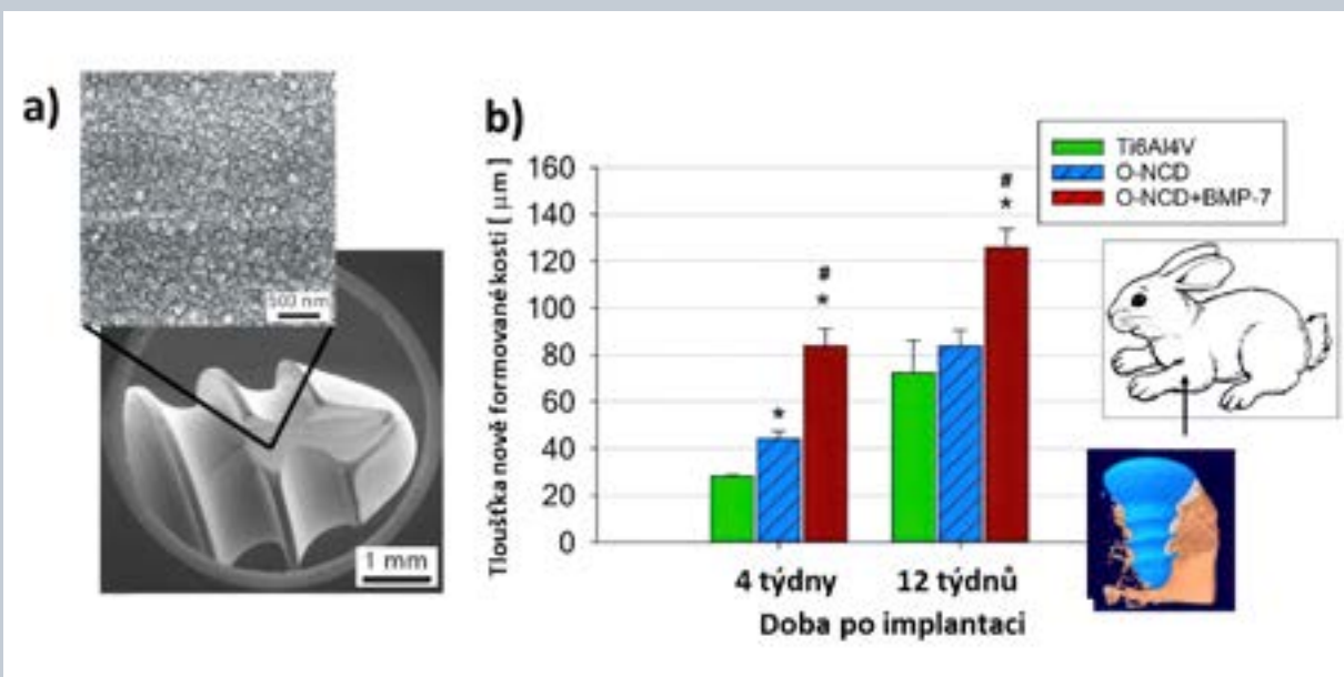
Obr. 2.3.2 a) Povrchová morfologie kortikálních vrutů pokrytých nanokrystalickým diamantem podél závitů. b) Schematické zobrazení místa implantace vrutu a kvantifikace nově vytvořené kosti ve střední části implantátu 4 a 12 týdnů po implantaci pro kontrolní vzorek (Ti6Al4V), kyslíkem terminovaný povrch NCD vrstvy (O-NCD), kyslíkem terminovaný povrch NCD s funkcionalizací molekulou BMP-7 (O-NCD + BMP-7) [6].
