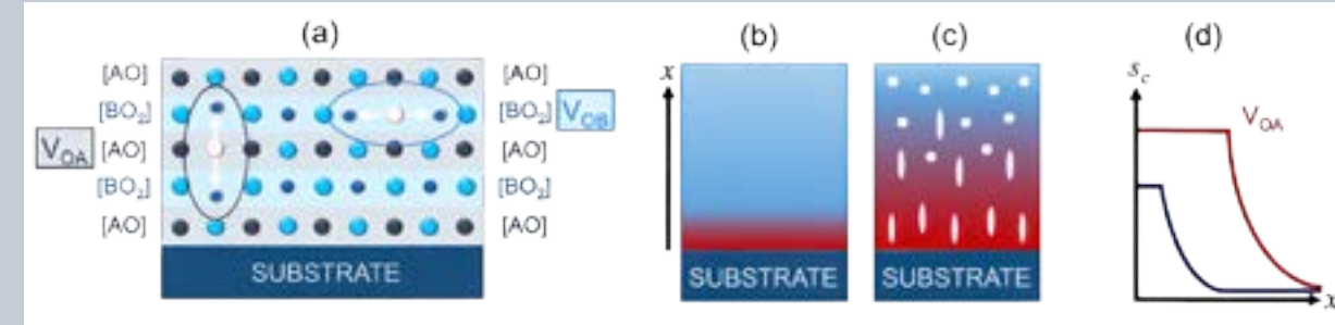
Obr. 2.4.2 Kyslíkové vakance v epitaxních \text{ABO}_3 perovskitových vrstvách.
