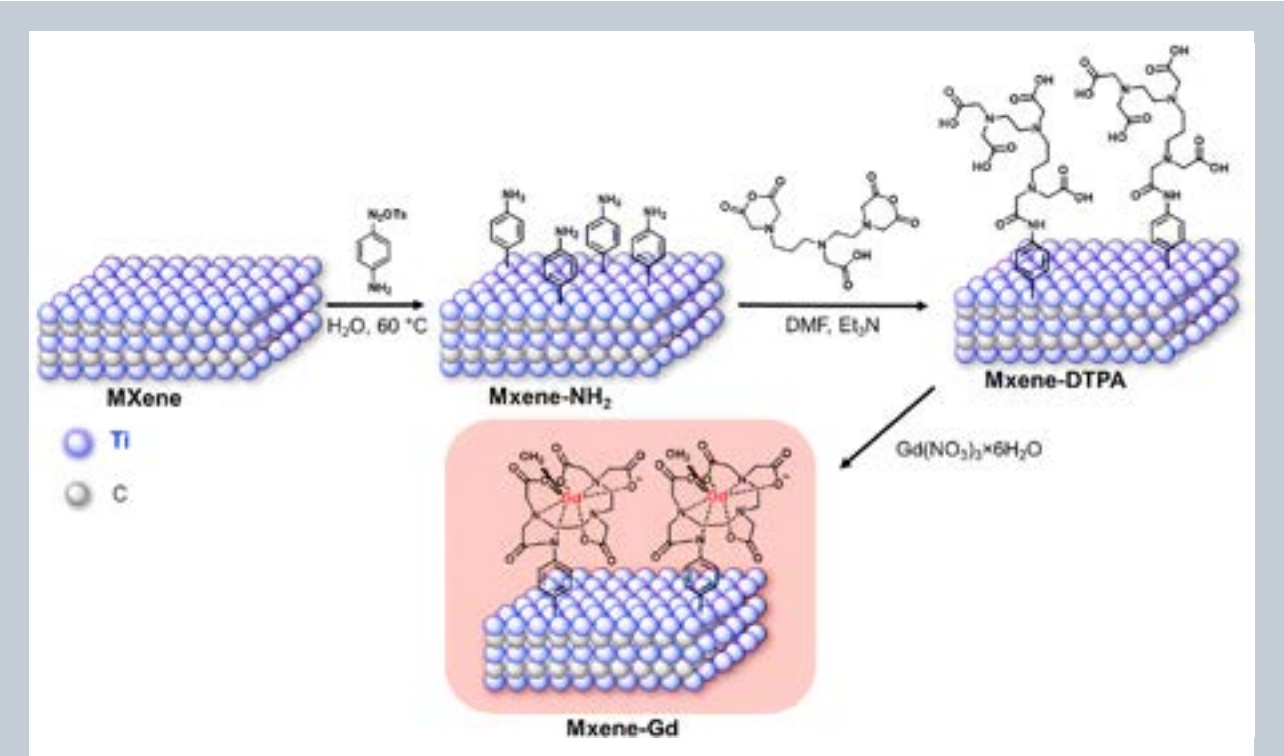
Obr. 2.4.4 Schematické znázornění funkcionalizace MXenových vloček v následujícím pořadí: modifikace pomocí diazoniové chemie pro připojení \text{-NH}_2 skupiny \text{MXene-NH}_2 \rightarrow MXen diethylentriaminpentaocetová kyselina (DTPA) a dále \rightarrow komplexování s \text{Gd}^{3+} ionty.
