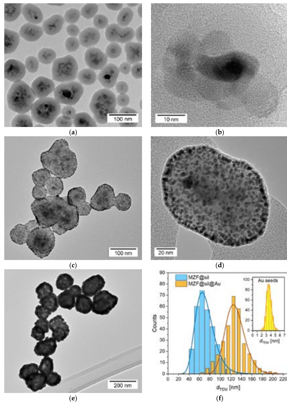
Obř. 2.3.5 Snímky z transmisní elektronové mikroskopie a distribuce velikostí nanočástic: (a) MZF@sil; (b) HRTEM detail magnetického jádra MZF@sil; (c, d) nanočástice MZF@sil dekorované zlatým koloidem; (e) finální produkt MZF@sil@Au; (f) histogramy velikostí MZF@sil a MZF@sil@Au s vložkou ukazující histogram jader Au na povrchu dekorovaného meziprojektu; model odpovídá lognormální distribuční funkci.
