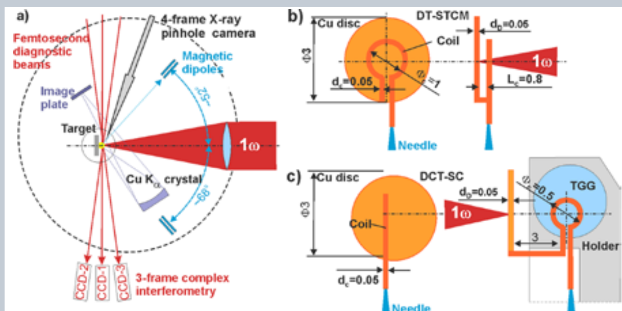
Obr. 2.5.5 Uspořádání interakčního experimentu [20]: (a) schéma umístění diagnostiky v experimentální komoře, (b) terč na bázi disk-cívka s jedním závitom pro vytvoření magnetizovaného plazmatu (DT-STCM), (c) terč DCT-SC upravený pro měření magnetického pole v cívkě pomocí Faradayova jevu v terbiu galiovém granátu (TGG).
