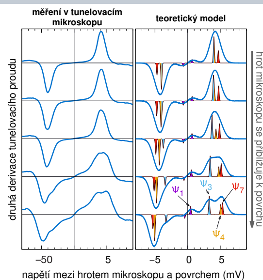
Obr. 2.2.5 Spektroskopické měření v řádkovacím tunelovacím mikroskopu s modifikovaným hrotem. Vlevo: schéma experimentu – na hrotu mikroskopu je umístěn spin se známými vlastnostmi, na povrchu je adsorbován neznámý spin. Uprostřed: změřený tunelovací proud pro různé vzdálenosti a různá napětí mezi hrotem a povrchem. Vpravo: výsledek teoretického modelu popisujícího neelastické tunelování skrz dva interagující spiny (čím blíže jsou, tím více interagují). Porovnáním teorie a experimentu je možné určit energie jednotlivých stavů ( \Psi ) systému dvou vázaných spinů, a odtud poté i vlastnosti původně neznámého spinu.
