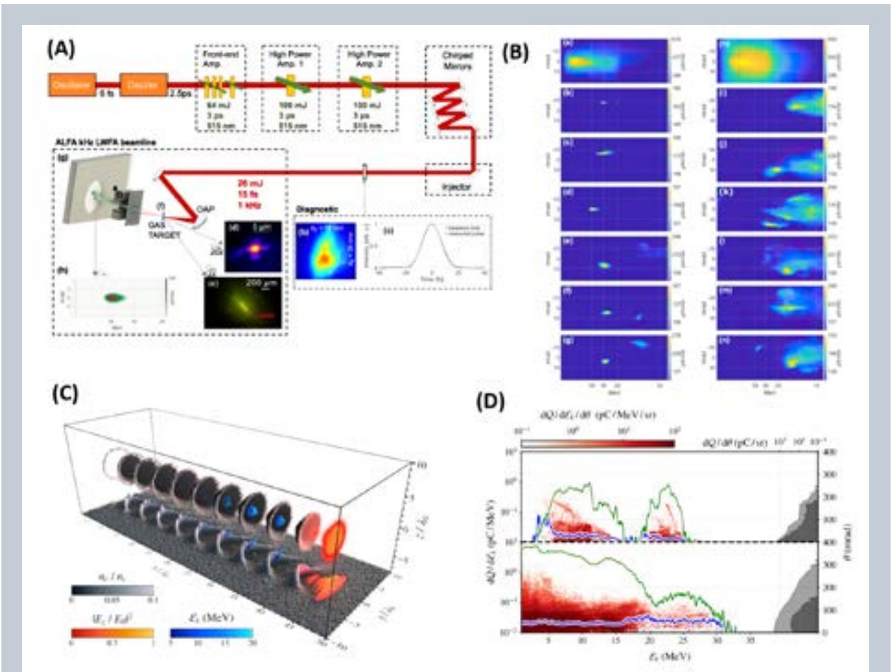
Obr. 2.6.1 Unikátní experiment, kde laserové pulzy s frekvencí 1 kHz urychlovaly 50 MeV elektrony. (A) Uspořádání experimentu, kde L1-Allegro laserový systém byl zaostřen na nadzvukový paprsek plynu. (B) Ukázka naměřených elektronových spekter. (C) 3D Simulace částice. (D) Simulované spektrum elektronového paprsku.
